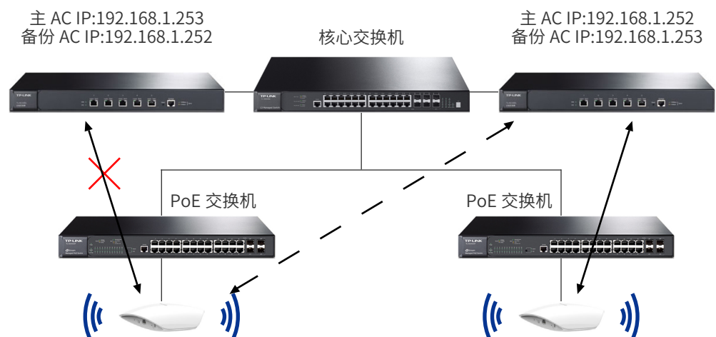
图 7-2 以 AC 为 DHCP 服务器网络拓扑图
