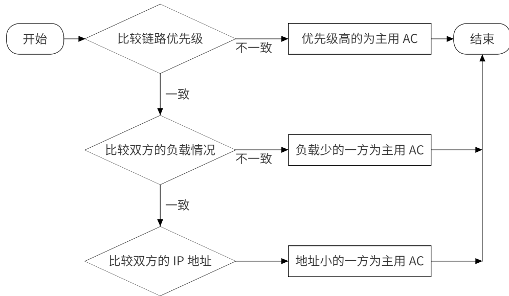
图 7-4 AP 选取主用 AC 规则流程图
