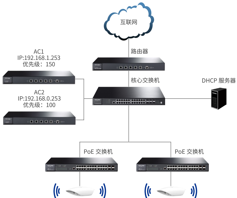
图 7-1 使用外部 DHCP 服务器网络拓扑图
